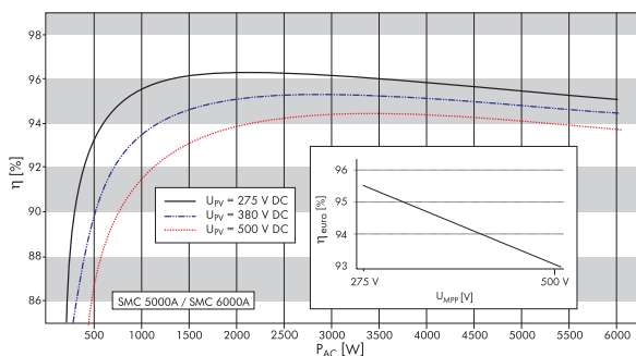
Wirkungsgradkurve
